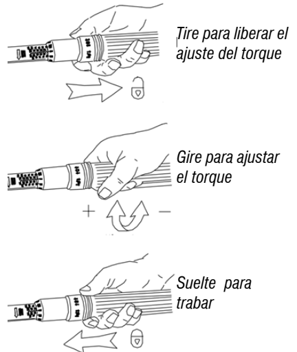
Fig. 2 – Ajuste de torque
