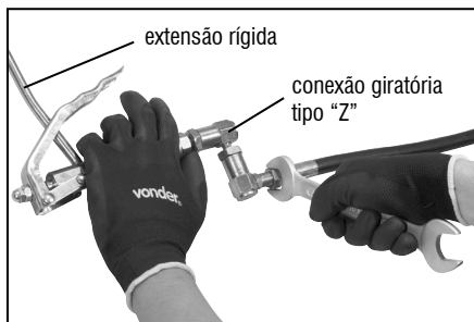
Figura 6 – Extensão rígida/conexão articulada
