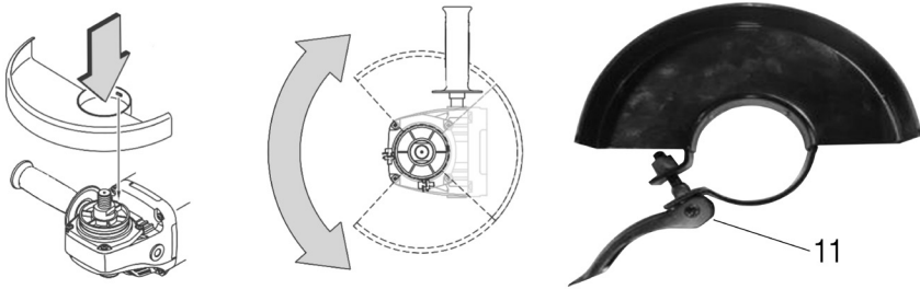
Figura 3 – Montagem e posicionamento da capa de proteção
