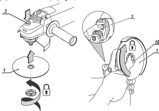
Figura 8 – Cambio del disco/Finalización de la sustitución
