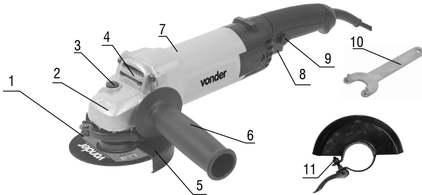
Figura 1 – Componentes de la Esmeriladora
