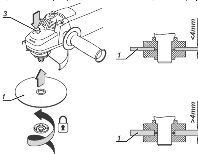
Figura 5 – Montaje del disco en la máquina
