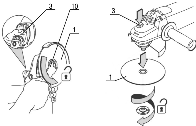
Figura 7 – Substitución del disco
