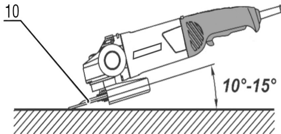
Figura 10 – Ângulo correto de esmerilhamento
