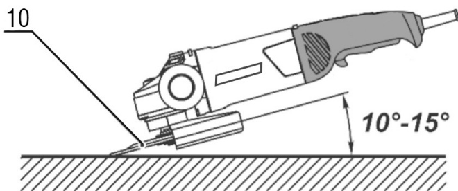
Figura 10 – Ángulo correcto de esmerilado
