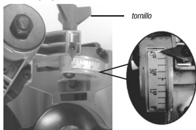
Fig. 16 – Posicionando el cabezal en el ángulo deseado
