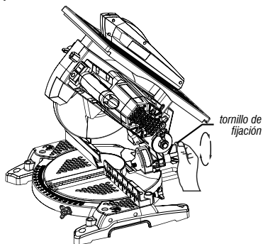
Fig. 15 – Liberando el ángulo del cabezal
