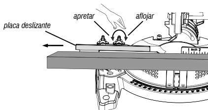
Fig. 14 – Reposicionando la placa deslizante
