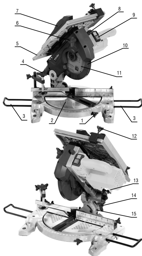
Fig. 1 – Componentes
