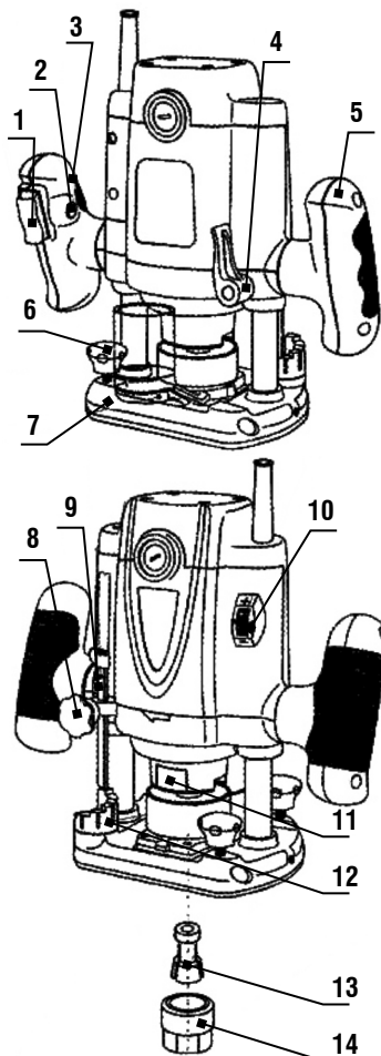
Fig. 1 – Componentes
