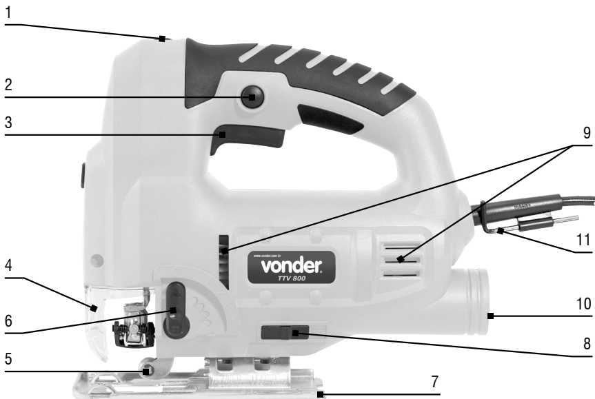
Figura 1 – Componentes da serra tico-tico
