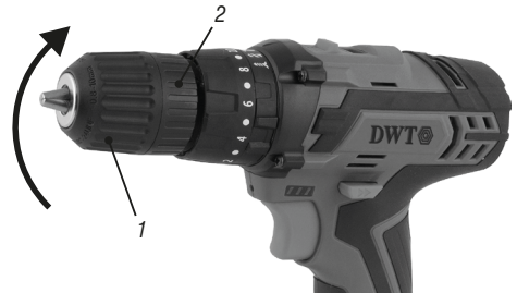
Fig. 3 – Apriete del mandril
