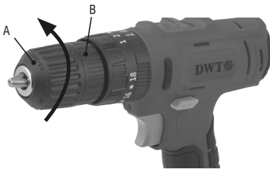
Fig. 7 – Apertura del mandril
