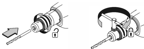
Fig. 2 – Desenho demonstrativo de aperto da broca no mandril
