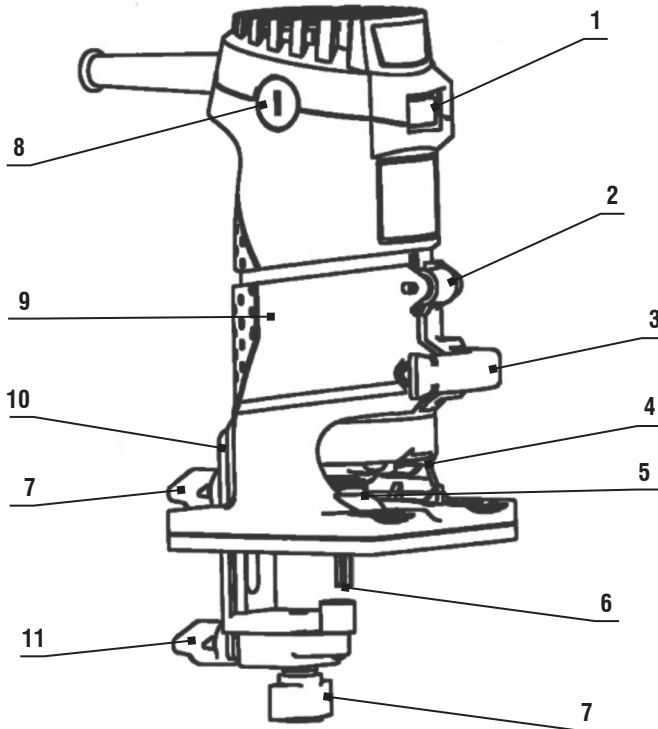
Figura 1 – Componentes da Tupia F-550
