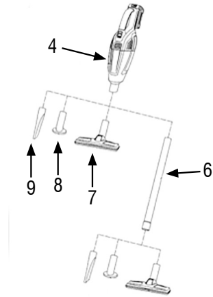
Fig. 2 – Combinação de montagem dos acessórios
