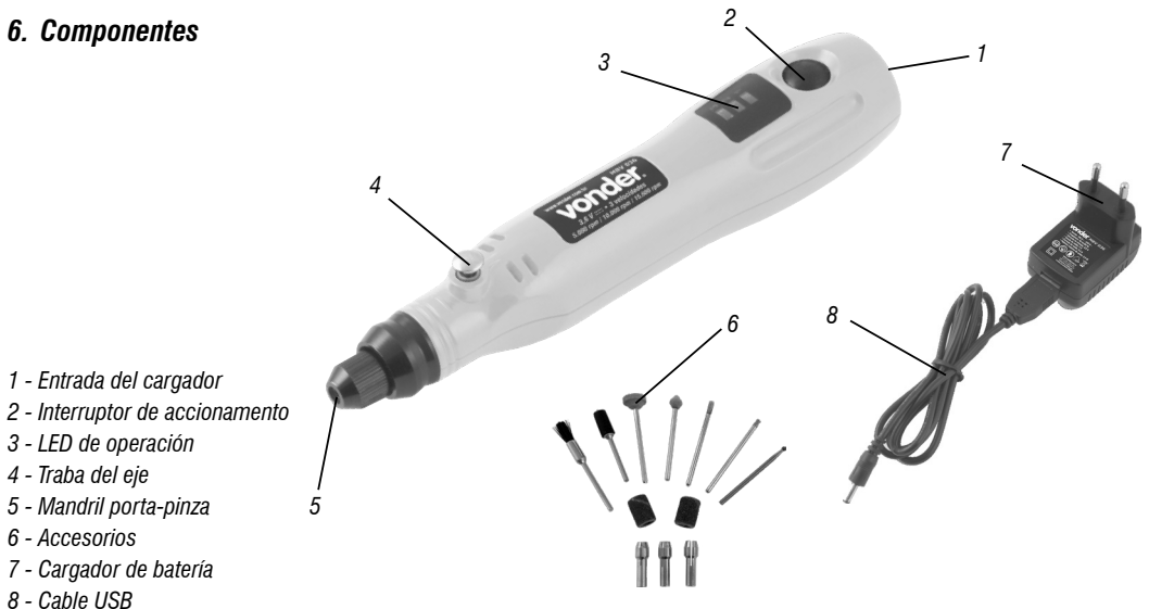
Fig. 1 – Componentes de la microrrectifica
