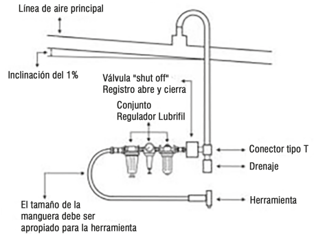
Fig. 4 – Diseño de la red de aire comprimido
