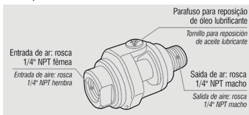
Fig. 2 – Minilubrificador
