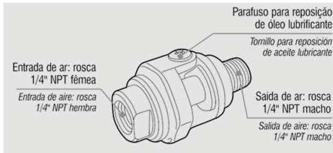
Fig. 2 – Minilubricador
