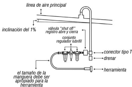
Fig. 2 – Proyecto de red de aire comprimido
