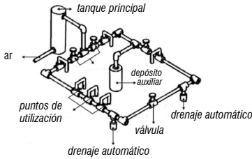
Fig. 1 – Red de aire comprimido
