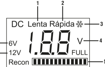
Figura 2 - Componentes del visor
