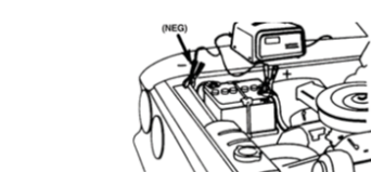
Figura 4 - Cargando la batería de un vehículo
