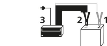
Figura 3 - Secuencia para conectar el cargador en la batería
