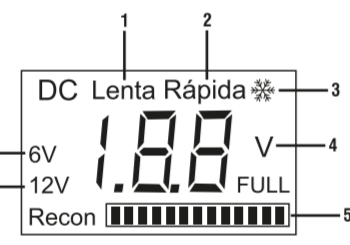
Figura 2 - Componentes do visor
