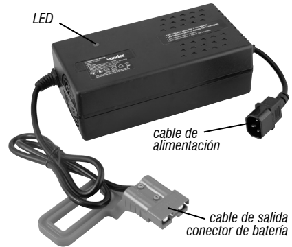
Fig. 1 – Componentes
