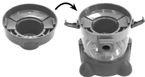
Fig. 5 – Tampa de proteção
