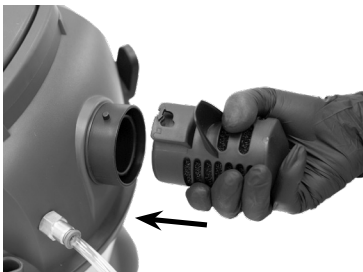
Fig. 13 – Insertando el silenciador
