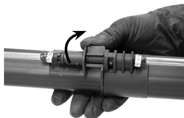
Fig. 15 – Posição fechada (para travar o encaixe)
