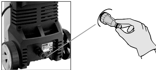
Figura 15 – Limpieza entrada de agua
