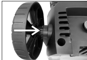
Figura 7 – Encaje de las ruedas
