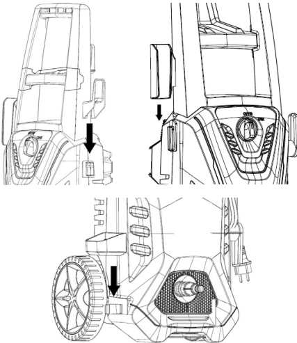
Fig. 3 – Montaje de los soportes
