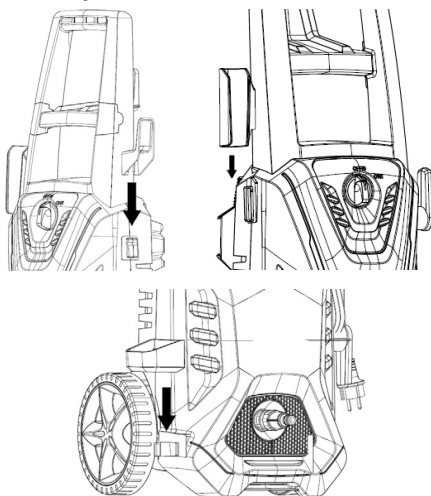
Fig. 3 – Montagem do suporte da pistola
