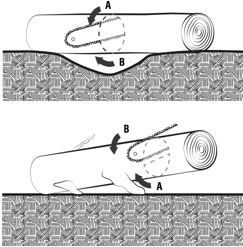
Fig. 17 – Corte sob tensão
