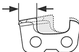
Fig. 23 – Dente com desgaste
