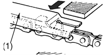
Fig. 25 – Rebaje del salto
