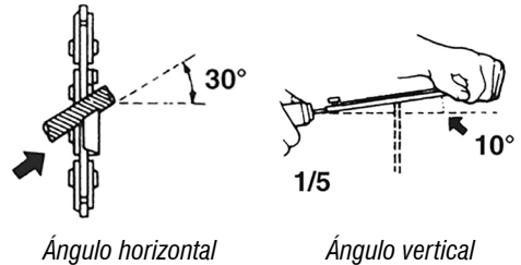
Fig. 21 – Ángulos de afilado
