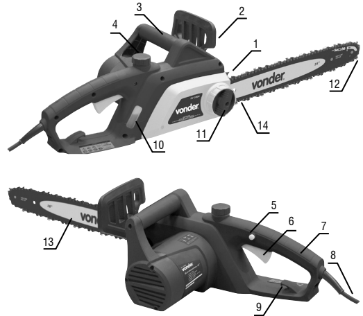
Fig. 2 – Componentes
