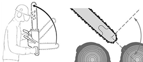
Fig. 1 – Rebote / Zona de riesgo de rebote
