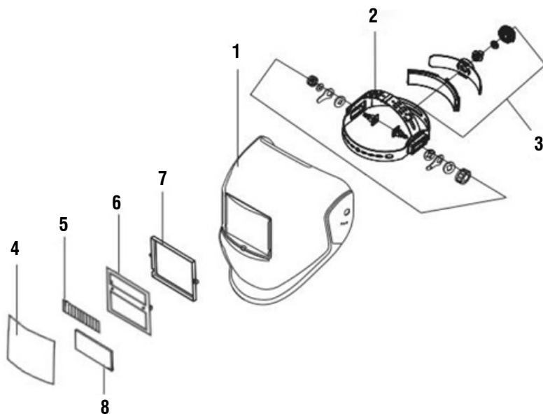
Fig. 1 – Componentes
