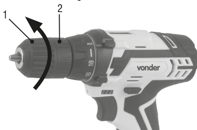
Fig. 3 – Abertura do mandril
