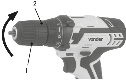
Fig. 4 – Apriete del mandril
