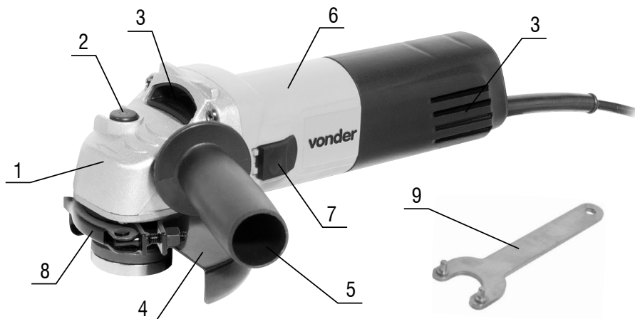
Figura 1 – Componentes da Esmerilhadeira
