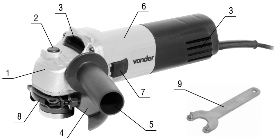
Figura 1 – Componentes de la Esmeriladora
