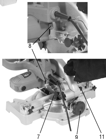
Fig. 1 – Componentes
