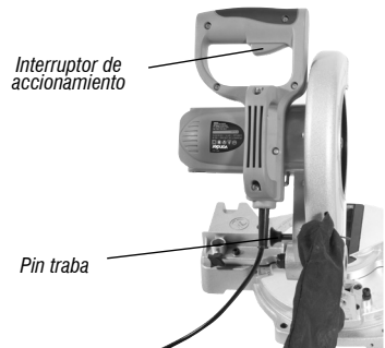
Fig. 3 – Movimiento de la cabeza de la máquina
