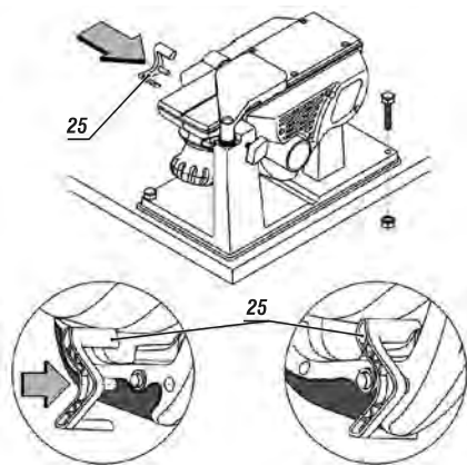
fig.15 - modo estacionário
