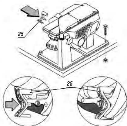
fig. 15 – modo estacionario
