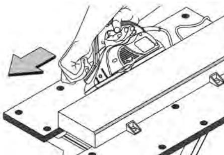
fig. 8 - chanfrando peças
