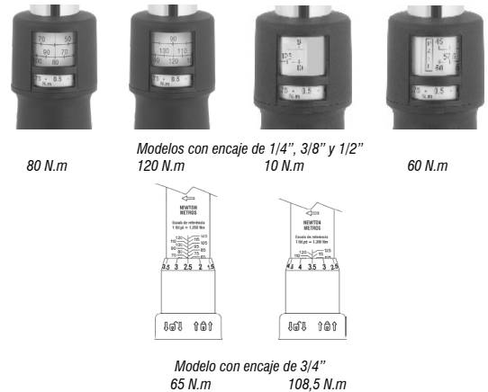
Figura 3 – Ejemplos de ajustes de torque
