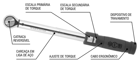
Figura 1 – Componentes modelos com encaixe 1/4", 3/8" e 1/2"
