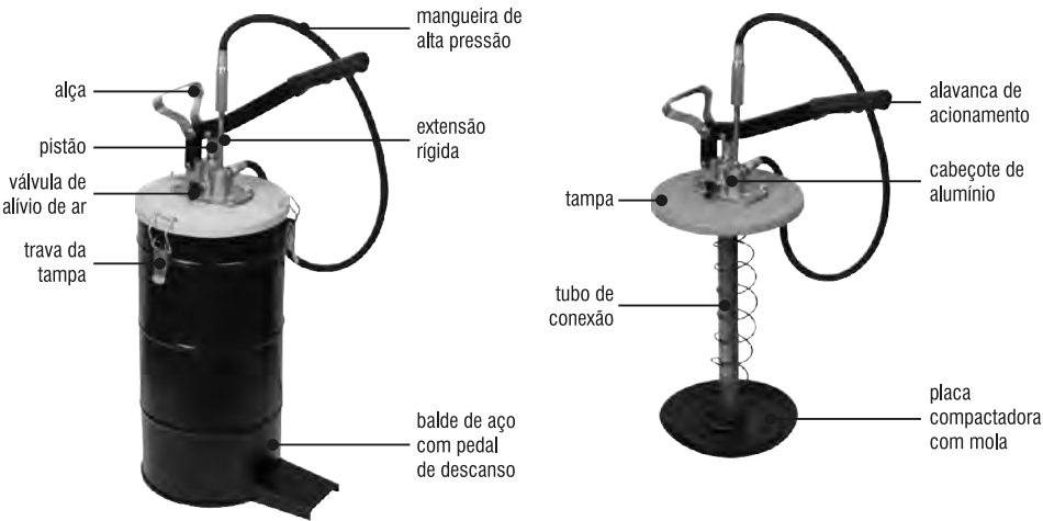
fig. 1 – balde para graxa
