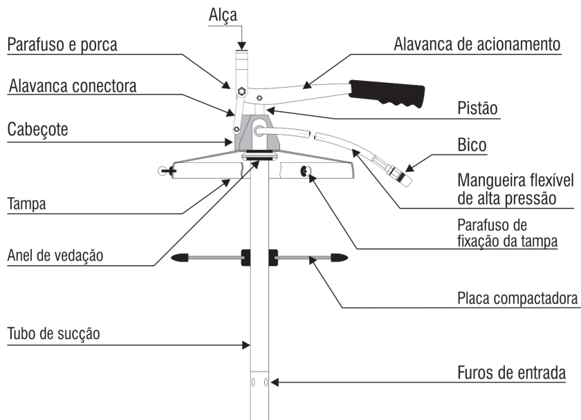
Fig. 1 – Tampa para Balde de Graxa TBV 0020 VONDER
