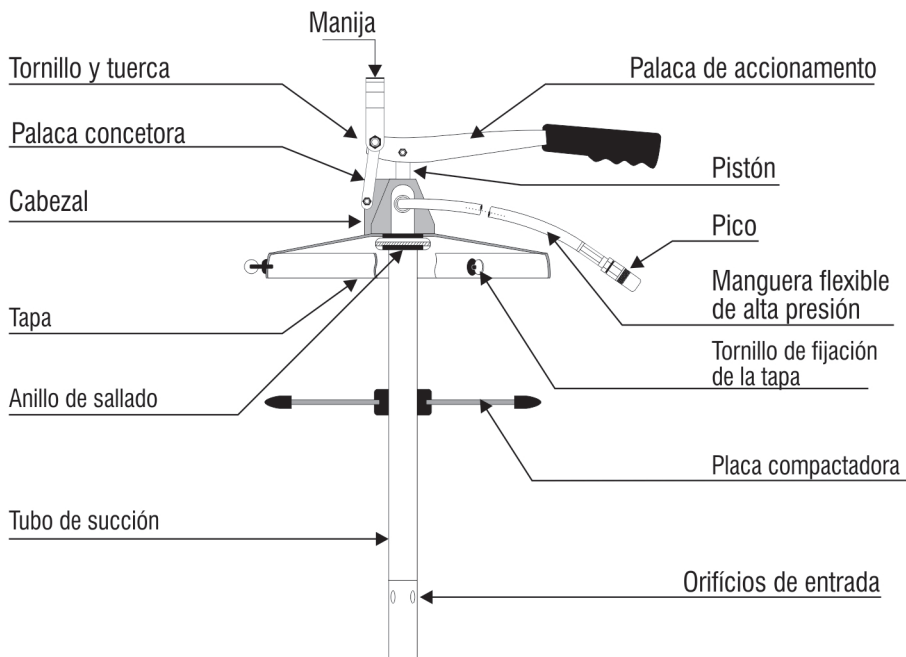
Fig. 1 – Tapa para Balde de Grasa TBV 0020 VONDER
