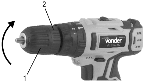
Fig. 4 – Apriete del mandril'
