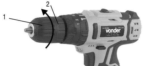
Fig. 3 – Apertura del mandril
