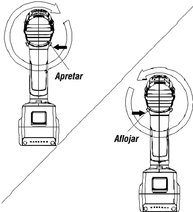
Fig. 4 – Sentido de rotación
