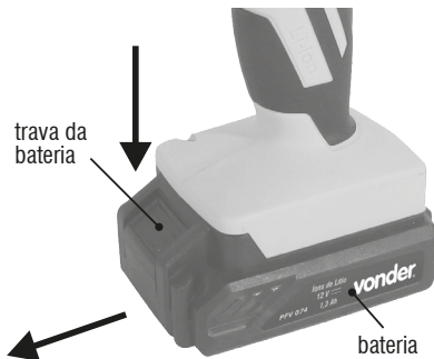
Fig. 9 – Retirando a bateria
