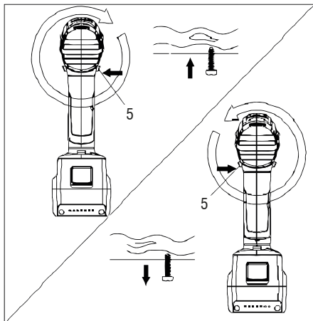
Fig. 8 – Sentido de rotación
