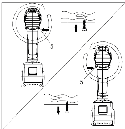
Fig. 8 – Sentido de rotação
