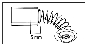
Fig. 4 – Deterioro del escobilla de carbón
