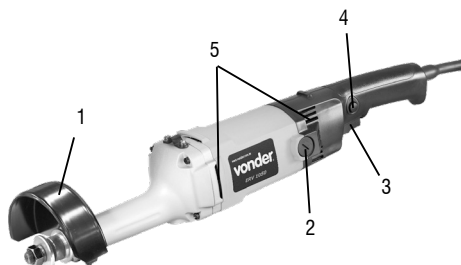
Fig. 1 – Componentes
