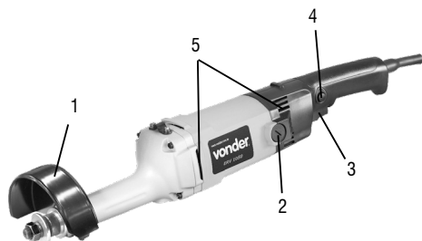
Fig. 1 – Componentes
