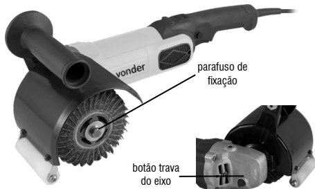
Fig. 4 – Orientação de instalação
