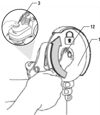
Fig. 6 – Montaje del disco en la herramienta
