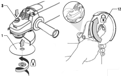
Fig. 8 – Trocando o disco
