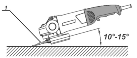
Fig. 11 – Ângulo correto de esmerilhamento
