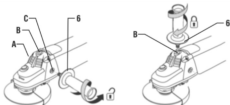
Fig. 2 – Cambio de posición del mango auxiliar
