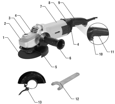
Fig. 1 – Componentes
