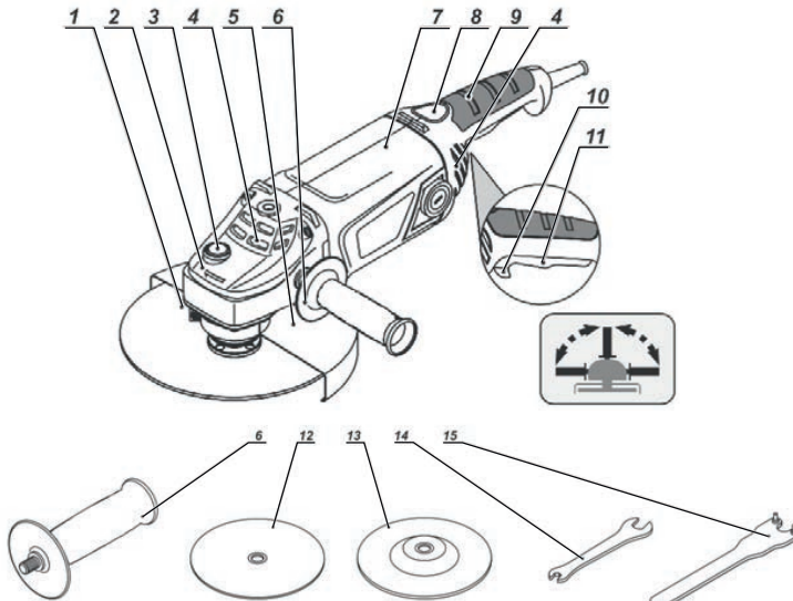
Figura 1 – Componentes de la Esmeriladora
