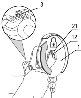
Fig. 6 – Montagem do disco na máquina
