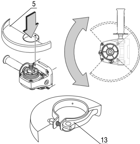
Fig. 3 – Montaje y posicionamiento de la capa de protección
