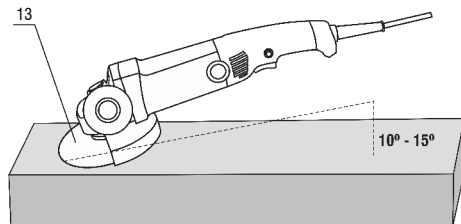
Fig. 8 – Ángulo correcto de esmerilado
