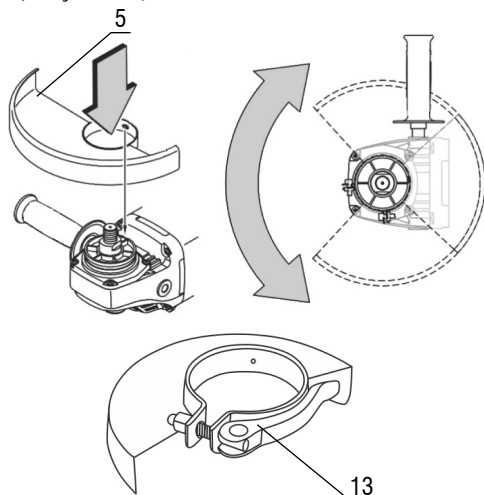
Fig. 3 – Montagem e posicionamento da capa de proteção
