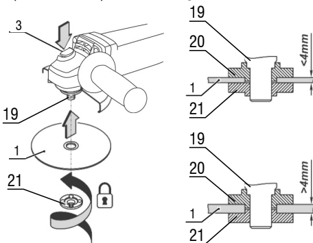
Fig. 5 – Montagem do disco na máquina
