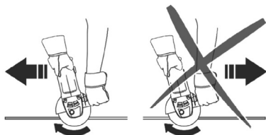
Fig. 7 – Dirección de corte correcto
