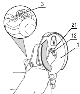
Fig. 6 – Montaje del disco en la máquina
