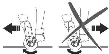
Fig. 7 – Sentido de corte correto
