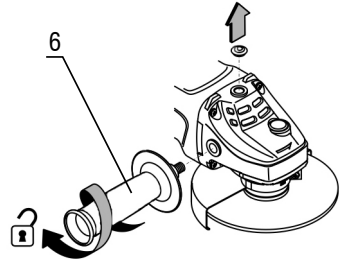
Fig. 2 – Montaje del puño auxiliar
