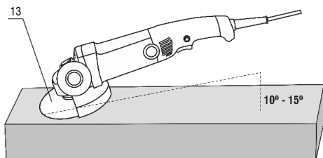
Fig. 8 – Ângulo correto de esmerilhamento
