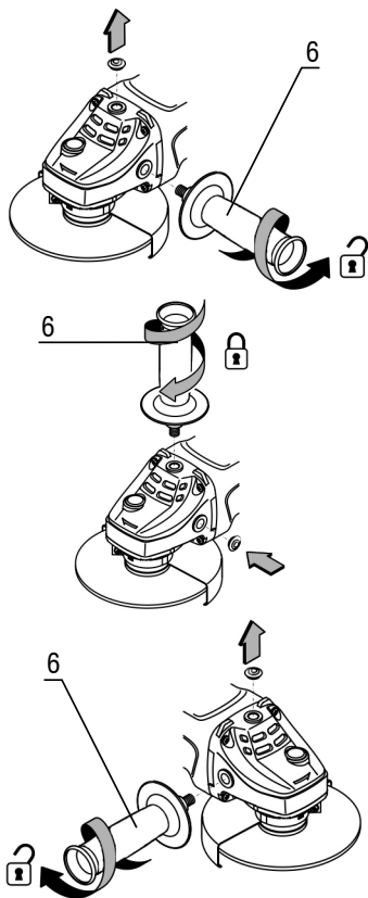
Fig. 2 – Montagem do punho auxiliar
