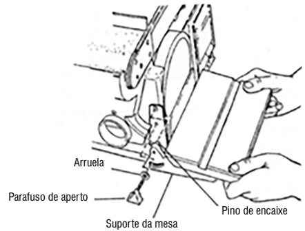
Fig. 3 – Montagem da mesa de trabalho
