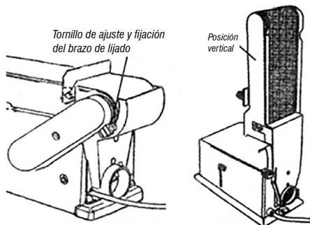
Fig. 10 – Ajuste del brazo de lijado
