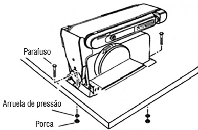
Fig. 2 – Instalando a Lixadeira Combinada na bancada
