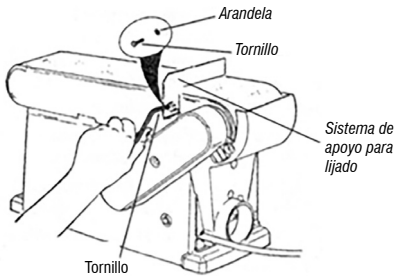
Fig. 4 – Instalación del sistema de apoyo para lijado
