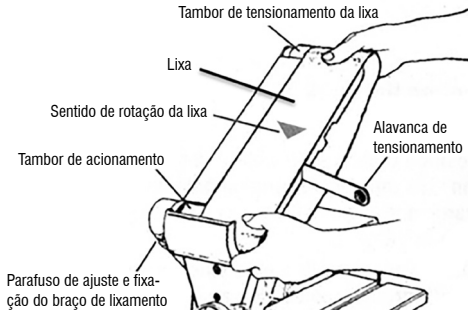
Fig. 7 – Trocando a lixa de cinta
