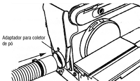
Fig. 5 – Entrada para coletor de pó
