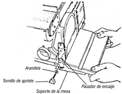
Fig. 3 – Montaje de la mesa de trabajo
