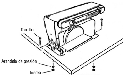
Fig. 2 – Instalación de la Lijadora Combinada en el banco
