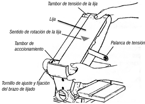
Fig. 7 – Cambiando la lija de cinta
