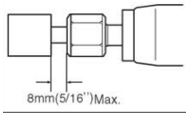
Figura 3 – Distância entre o porta-pinça e o acessório
