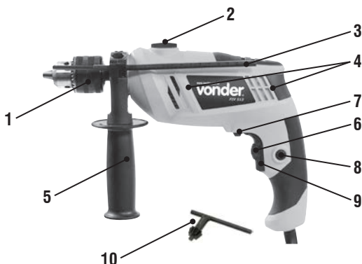
Figura 1 – Componentes del taladro
