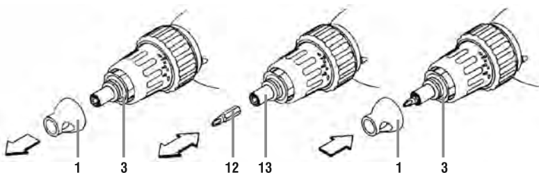
fig. 1 - instalação e substituição do bits / ponteira
