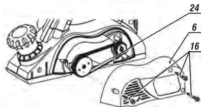
fig. 14 - substituição da correia
