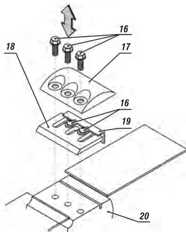
fig. 10 – sustitución de las cuchillas
