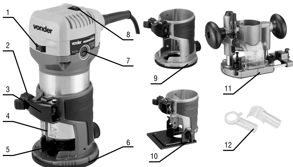
Fig. 1 – Componentes
