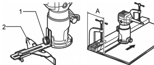
Fig. 9 – Fijación de la guía
