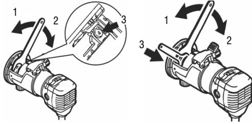
Fig. 5 – Instalando ou removendo a fresa
