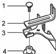
Fig. 8 – Montaje de la guía
