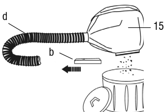
Fig. 6 – Vaciando el saco de polvo
