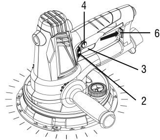
Fig. 7 – Encendiendo y apagando la máquina
