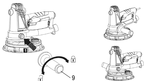
Fig. 2 – Montando el puño auxiliar
