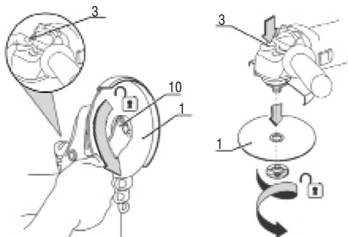
Figura 7 – Substituição do disco
