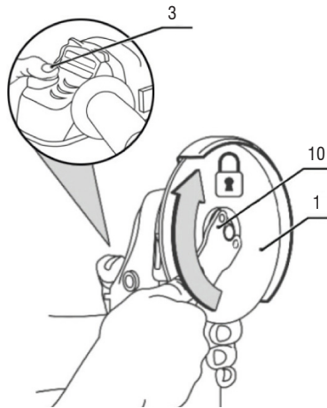
Figura 6 – Montaje del disco en la máquina
