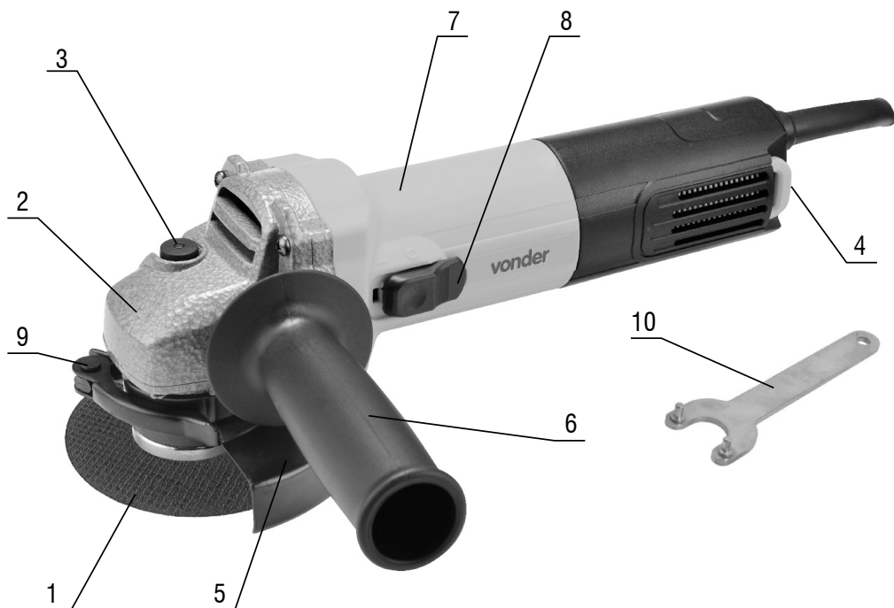
Figura 1 – Componentes da Esmerilhadeira
