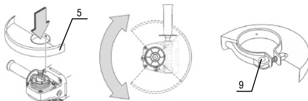
Figura 3 – Montagem e posicionamento da capa de proteção
