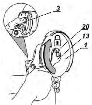
Fig. 6 – Montagem do disco na máquina
