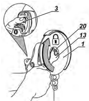
Fig. 6 – Montaje del disco en la máquina
