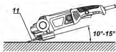
Fig. 10 – Ángulo correcto de esmerilado
