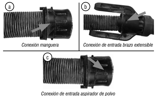
Fig. 3 – Conexión de entrada aspirador de polvo
