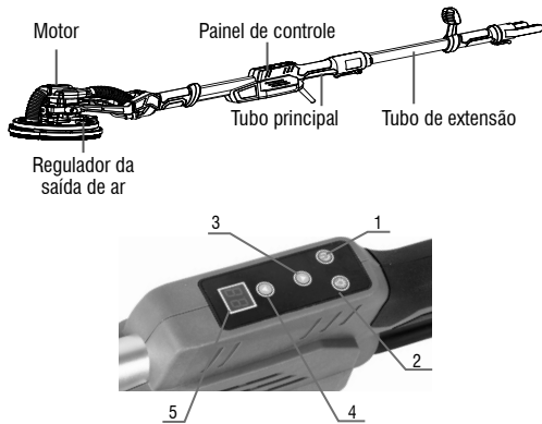
Fig. 1 – Componentes
