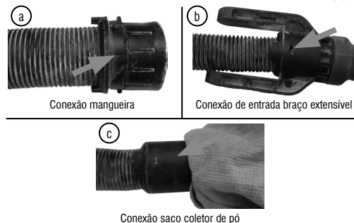
Fig. 2 – Conexão saco coletor de pó
