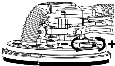
Fig. 8 – Ajustar la potencia de succión
