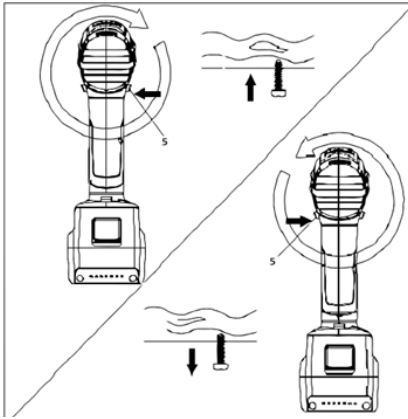
Fig. 4 – Sentido de rotación
