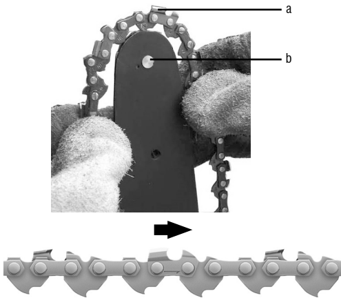
Fig. 4 – Instalación de la cadena de corte
