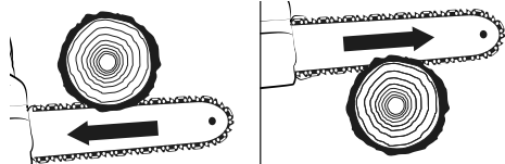
Fig. 20 – Segurança no corte transversal
