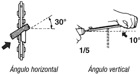
Fig. 25 – Ángulos de afilado
