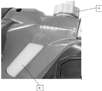
Fig. 16 – Tapa del tanque y visor de aceite
