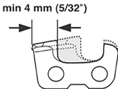
Fig. 27 – Diente con desgaste
