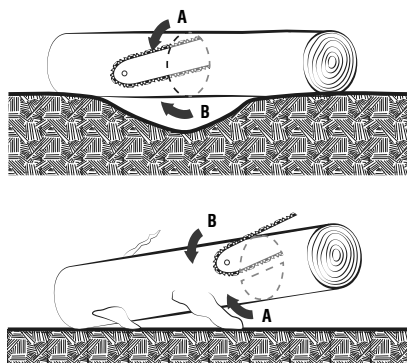
Fig. 21 – Corte sob tensão
