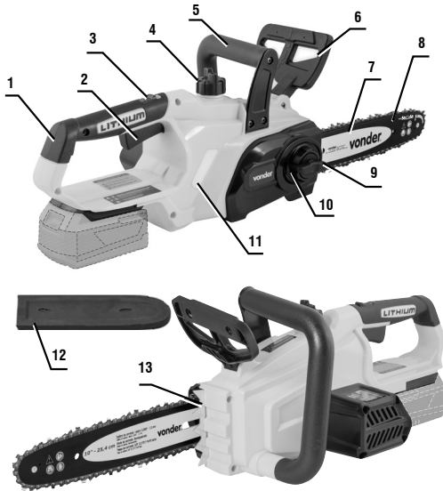
Fig. 2 – Componentes
