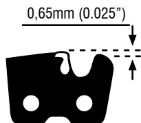
Fig. 28 – Salto de corte
