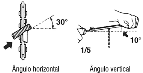
Fig. 25 – Ângulos de afiação
