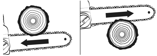
Fig. 20 – Seguridad en el corte transversal
