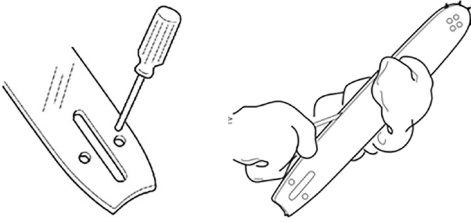
Fig. 18 – Limpieza del agujero de lubricación y canal del sable
