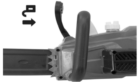
Fig. 15 – Liberación manual del freno
