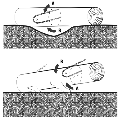
Fig. 21 – Corte bajo tensión
