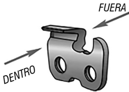
Fig. 26 – Posición de los dientes de corte
