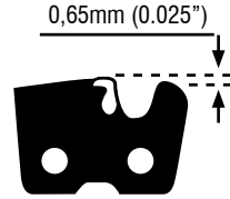
Fig. 28 – Salto de corte
