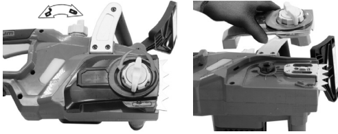
Fig. 3 – Removiendo la cubierta del sable de la cadena
