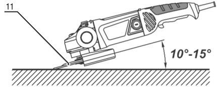
Fig. 10 – Ángulo correcto de esmerilado
