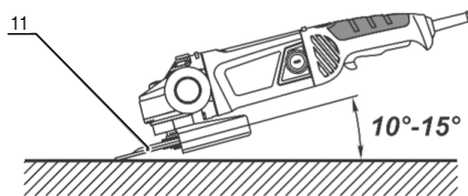
Fig. 10 – Ângulo correto de esmerilhamento
