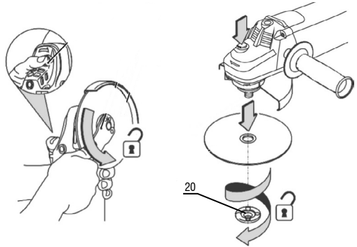
Fig. 7 – Substituição do disco
