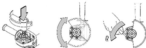
Fig. 3 – Montagem e posicionamento da capa de proteção
