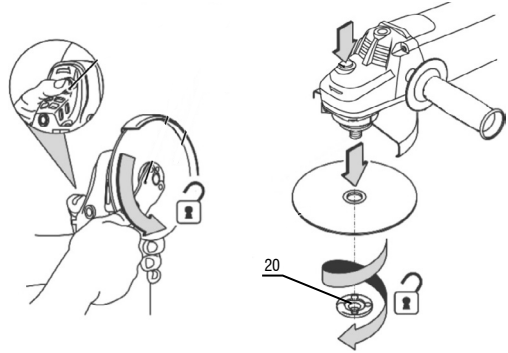
Fig. 7 – Sustitución del disco
