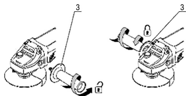
Fig. 2 – Montaje del puño auxiliar
