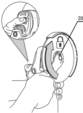
Fig. 6 – Montagem do disco na máquina
