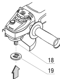
Fig. 4 – Montaje de accesorio en la máquina
